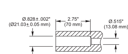
Section A-A (16X)
