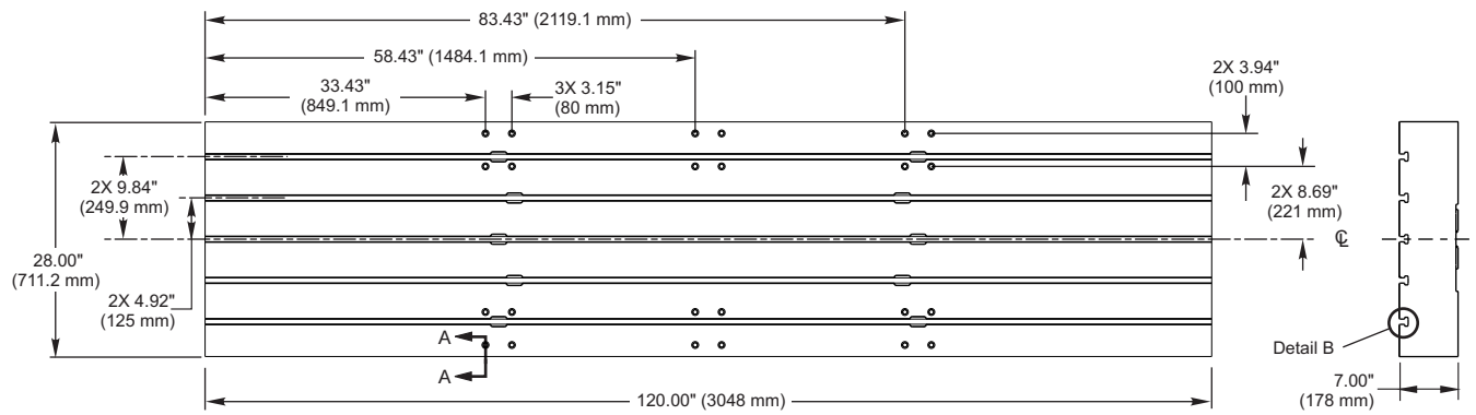
VF-11 Table Dimensions
