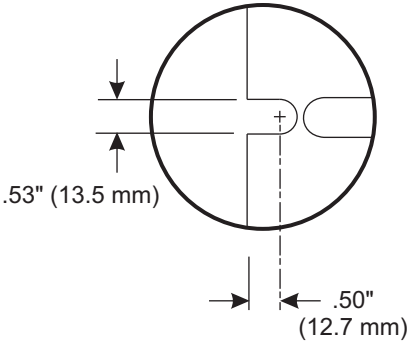
Tie-Down Slots
